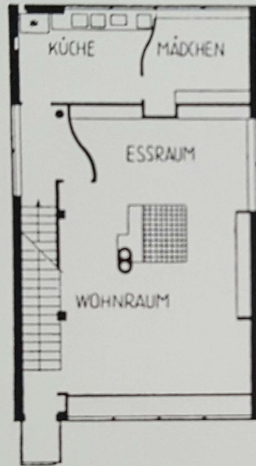
Wohngeschoß
